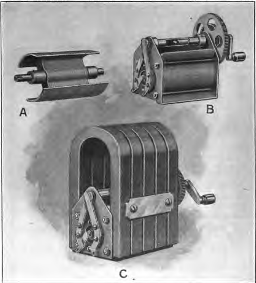
FIG. 72.—Magneto generator.
